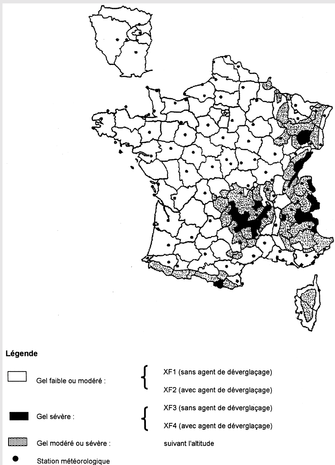
Figure NA.2 — Carte des zones de gel en France
