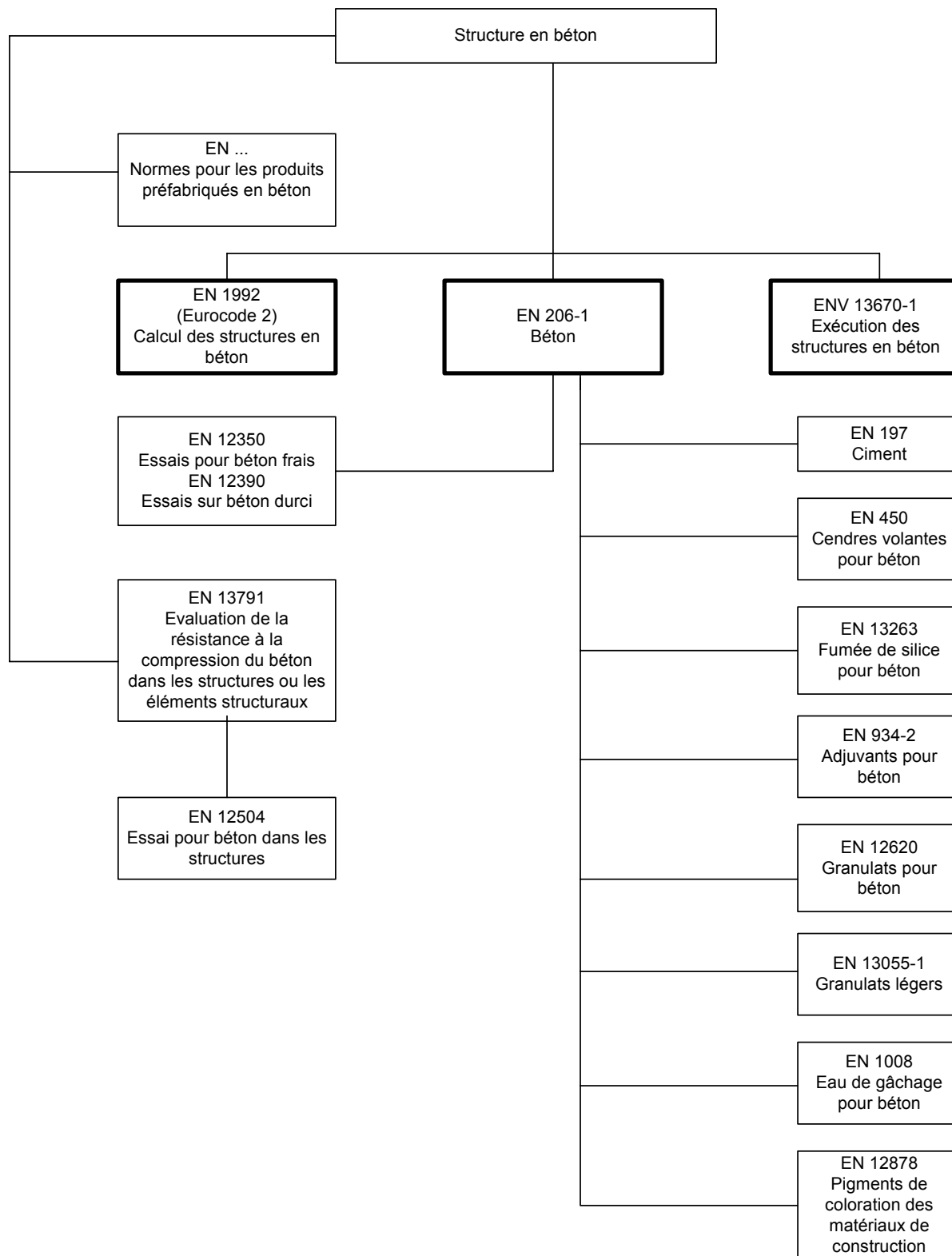
Figure 1 — Relations entre EN 206-1 et les normes pour la conception et l'exécution, ainsi que les normes relatives aux constituants et les normes d'essais
