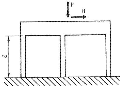
figure sans légende dans: E.7.3,13 cas où l'on peut se ramener à un poteau isostatique
