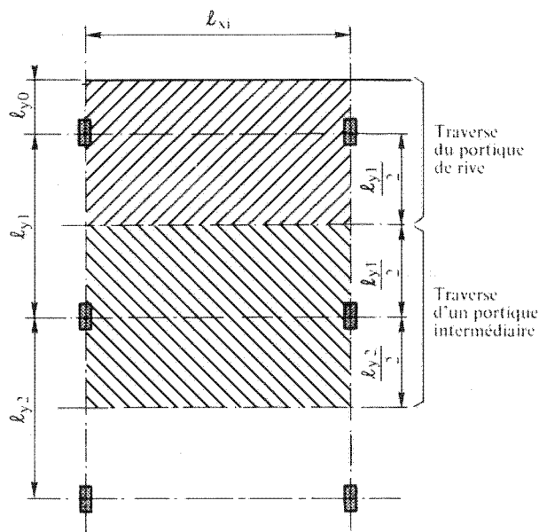
figure sans légende dans: E.4.1,2 méthode générale de calcul des sollicitations
