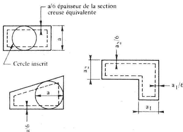
figure sans légende dans: A.5.4,22 sections pleines
