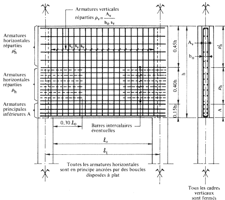
Figure 5 paroi fléchie à une travée h < l_t ( l_t = \min(l_d; 1, 15 l_o) )
