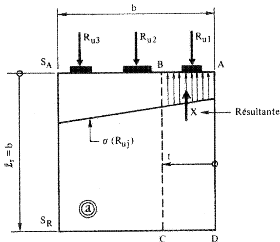
figure sans légende dans: E.8.2,4 justification vis-à-vis de l'équilibre général de diffusion pure ...
