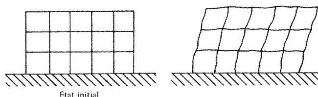
figure sans légende dans: E.7.3,22 ossatures à noeuds déplaçables
