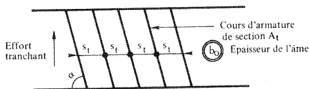
figure sans légende dans: A.5.1,22 section minimale d'armatures d'âme
