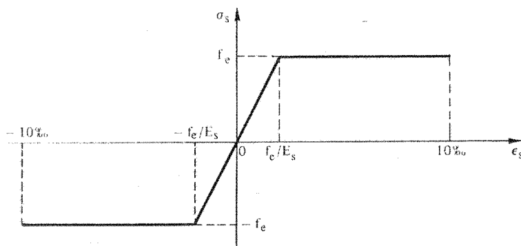
figure sans légende dans: A.2.2,2 diagramme déformations-contraintes
