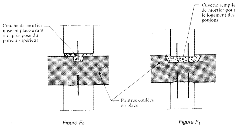
figure sans légende dans: B.8.6,22 liaison entre poteaux superposés
