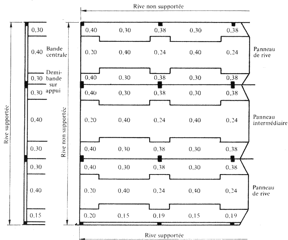
figure sans légende dans: E.4.8,24 cas des porte-à-faux
