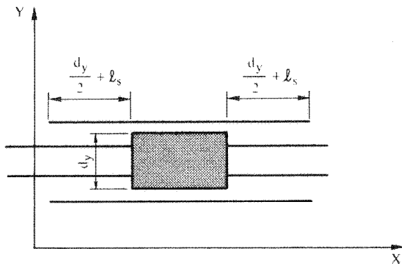
figure sans légende dans: E.4.8,4 trémies dans la dalle
