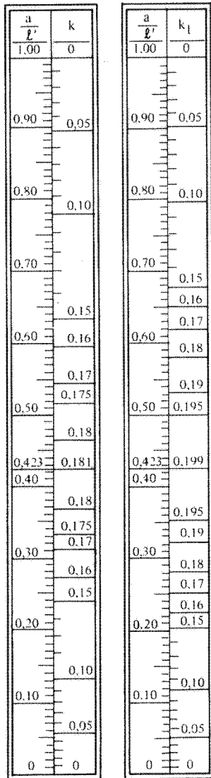
figure sans légende dans: E.2.2,1 moments d'appuis
