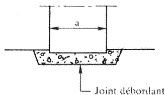
figure sans légende dans: B.8.6,22 liaison entre poteaux superposés
