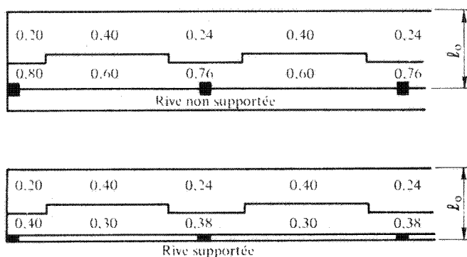
figure sans légende dans: E.4.8,24 cas des porte-à-faux
