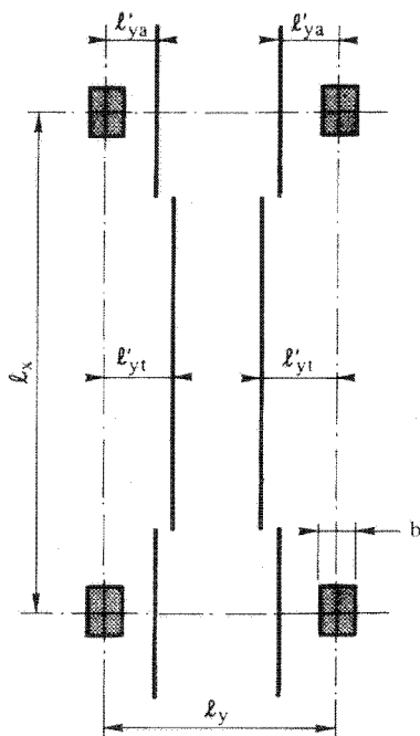
figure sans légende dans: E.4.8,22 division des panneaux en bandes
