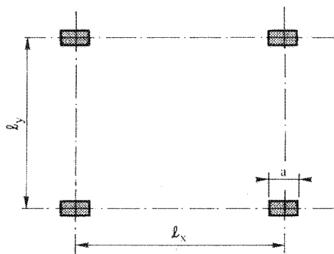
figure sans légende dans: E.4.8,21 moments fléchissants à prendre en compte dans les panneaux
