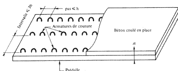
figure sans légende dans: B.7.6,23 justifications sous sollicitations tangentes
