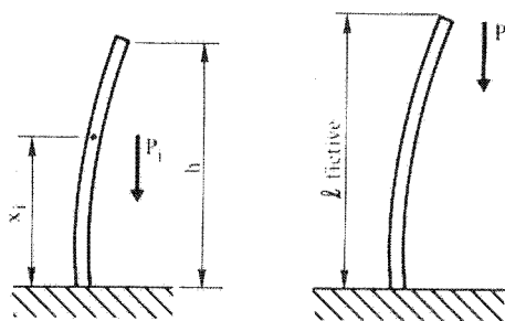
figure sans légende dans: E.7.2,2 mât soumis à des charges telles que l'effort normal ne soit pas ...
