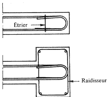
figure sans légende dans: E.5.4,11 parois fléchies reposant sur deux appuis
