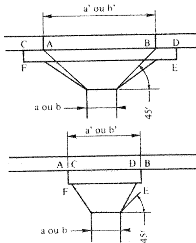
figure sans légende dans: E.4.0,3 chapiteaux
