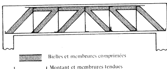
figure sans légende dans: B.6.8,5 poutre justifiée par la méthode du treillis
