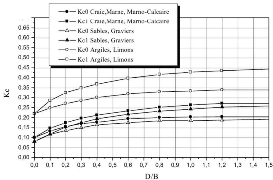
Figure 2.8. Valeurs du facteur de portance pénétrométrique K_c selon le DTU 13-12 [8]
