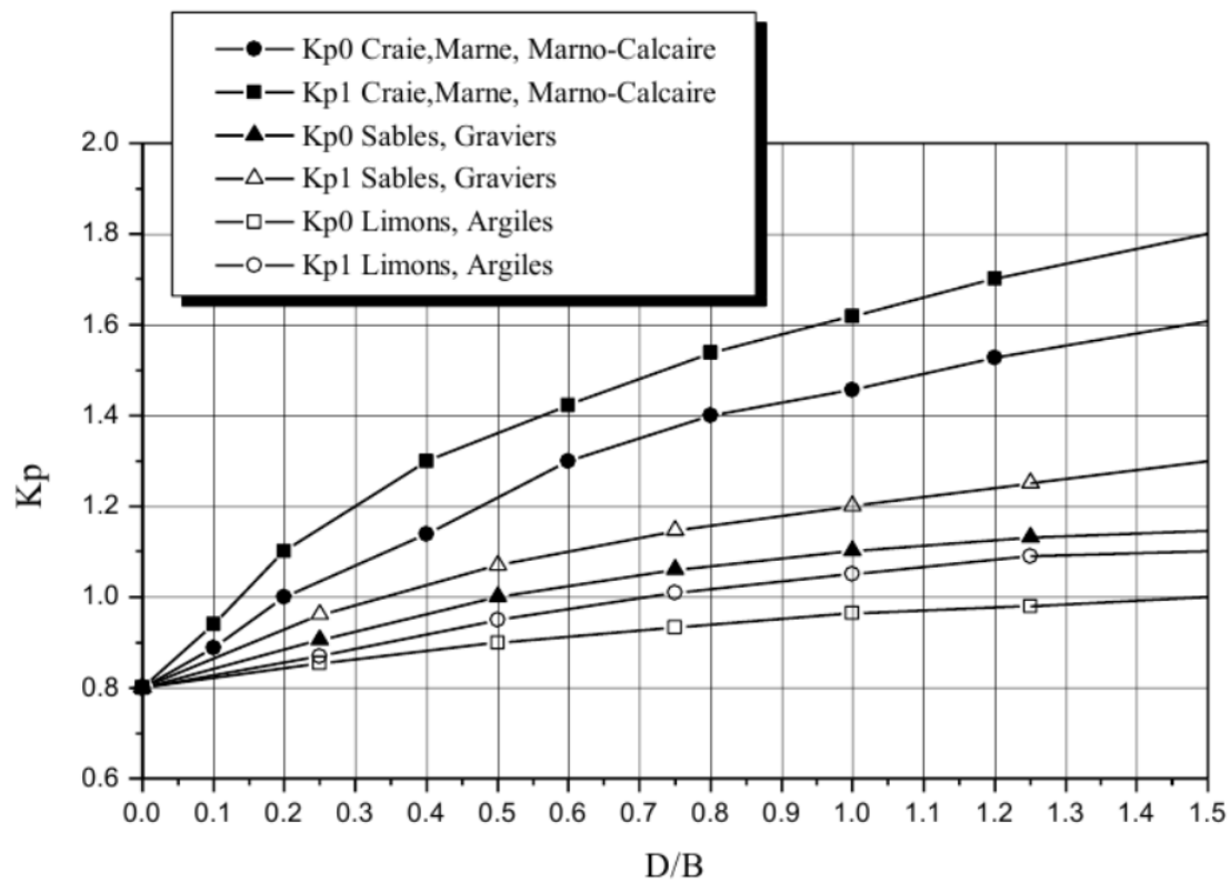
Figure 2.7. Facteur de portance pressiométrique selon le DTU 13.12 [8]
