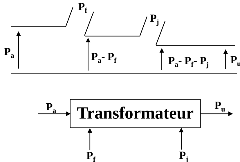
Figure .... Arbre des puissances.
