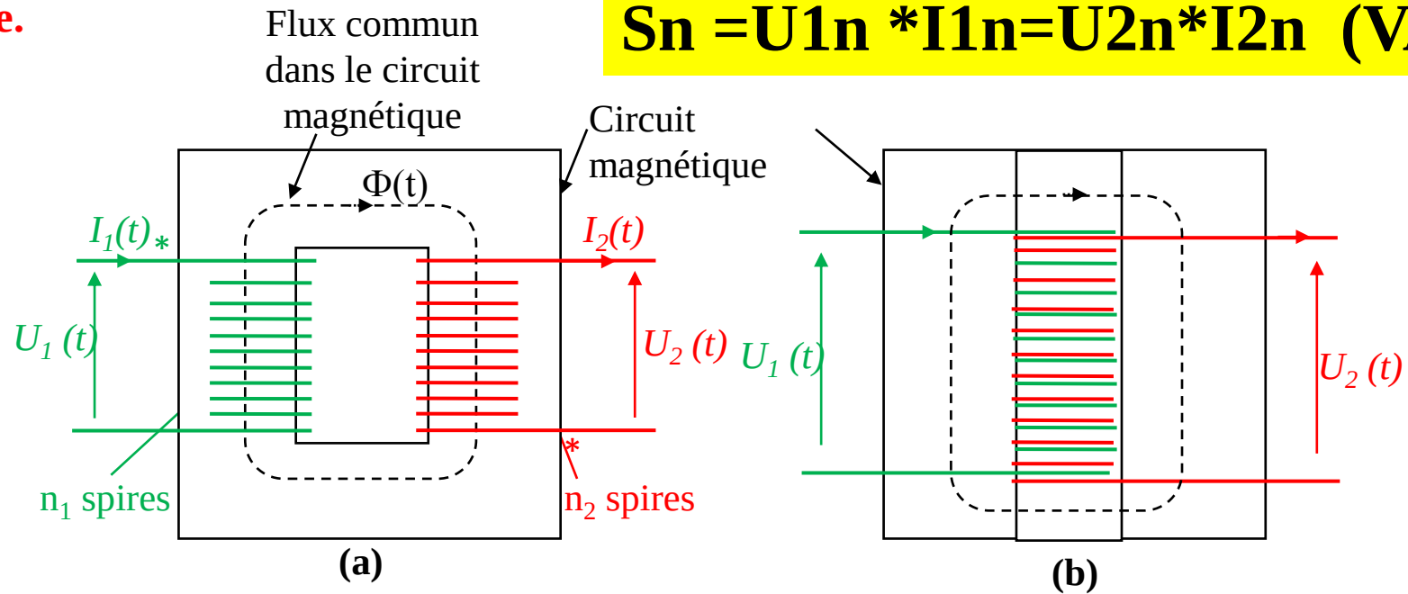
Figure .2. Constitution d'un transformateur monophasé.
