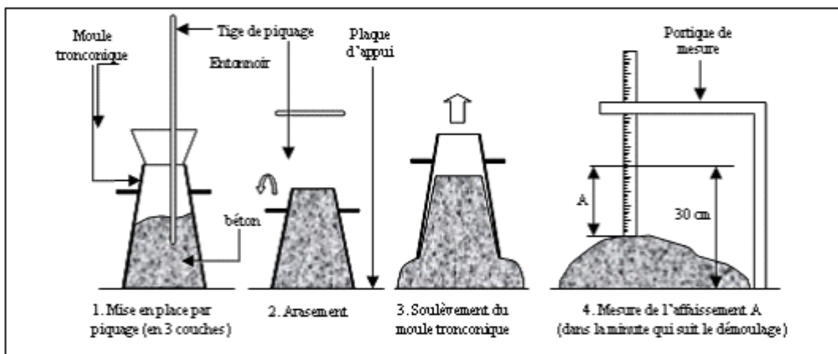
Figure 1-Cône d'abrams
