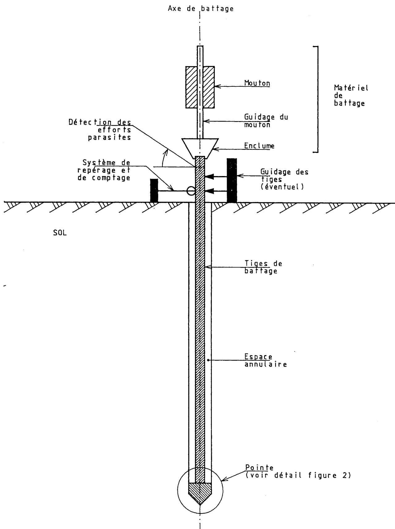
Figure 1 — Pénétrömètre dynamique PDB
