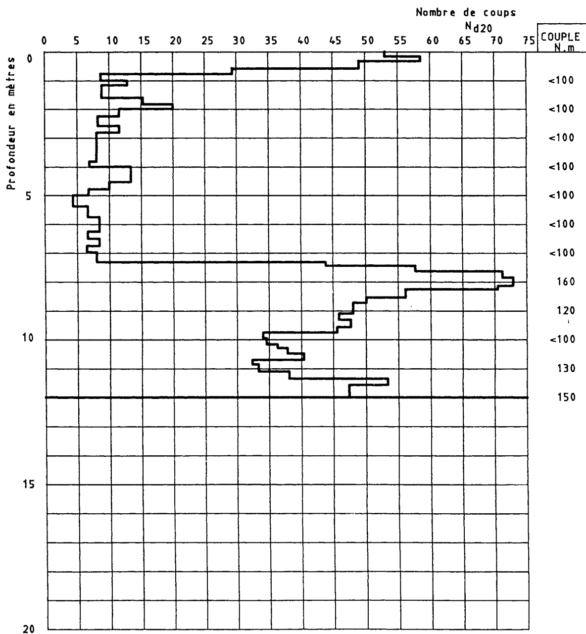
Figure B.1 — Procès-verbal du sondage au pénétromètre dynamique PDB
