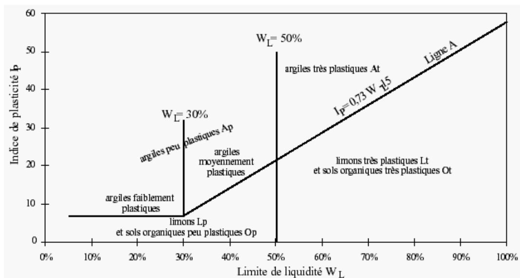
Fig. 1 : Classification des sols fins (diagrammes de Casagrande).
