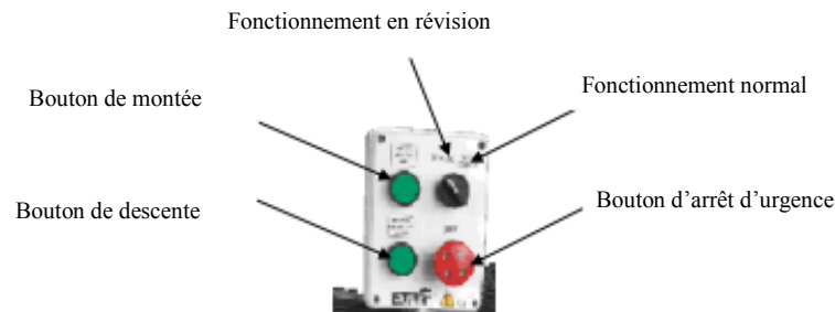
Figure (V.13) : Boîte d'inspection.
