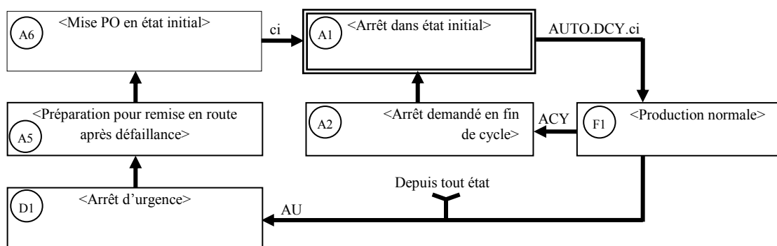
Figure (IV.11) : GEMMA d'une machine avec arrêt d'urgence.
