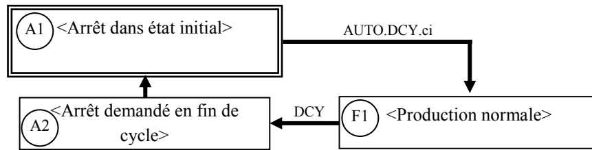
Figure (IV.7) : GEMMA minimal d'une machine automatique.
