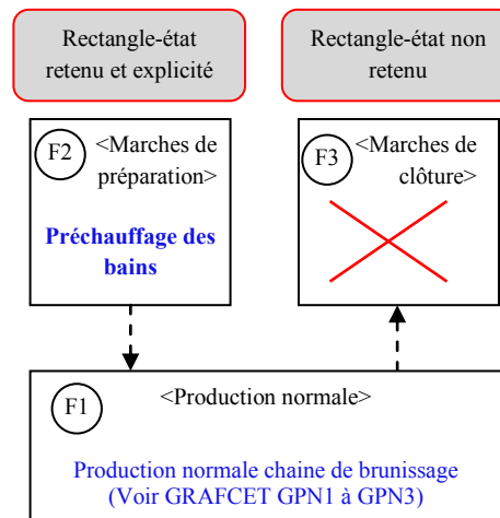
Figure (IV.4) : Le rectangle-état F2 est retenu, le rectangle-état F3 n'est pas retenu.
