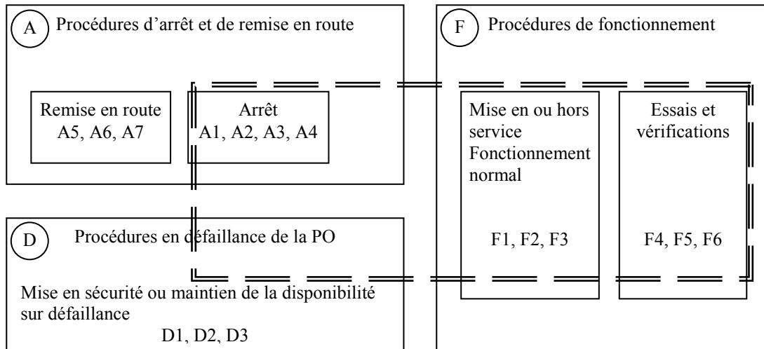
Figure (IV.1) : Les familles et les sous-familles de procédures.
