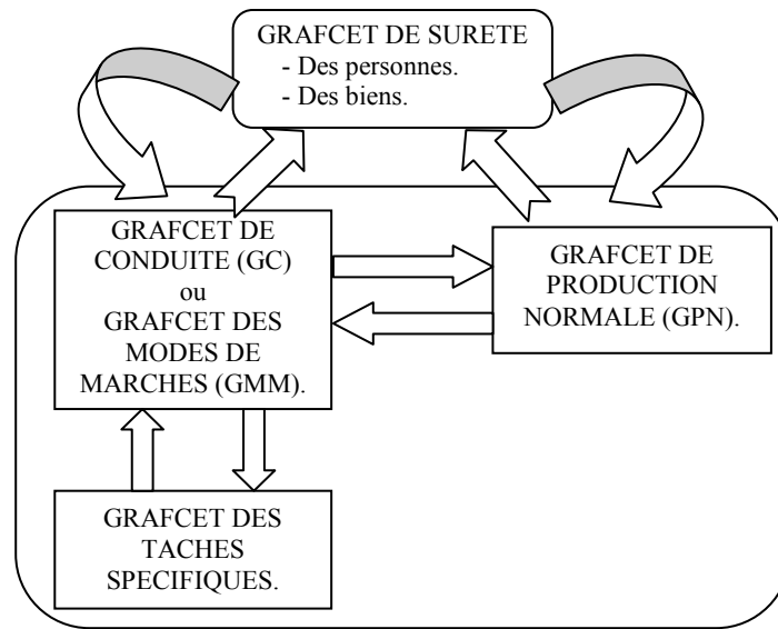
Figure (IV.16) : Réalisation de GRAFCET a partir du GEMMA.
