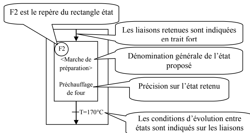
Figure (IV.2) : Représentation d'un rectangle-état.
