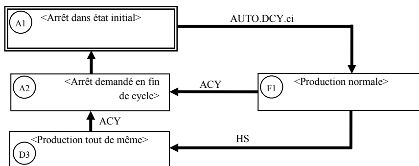
Figure (IV.13) : GEMMA d'une machine avec production tout de même.
