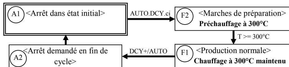
Figure (IV.8) : GEMMA d'une machine automatique ou semi-automatique exigeant une marche de préparation.
