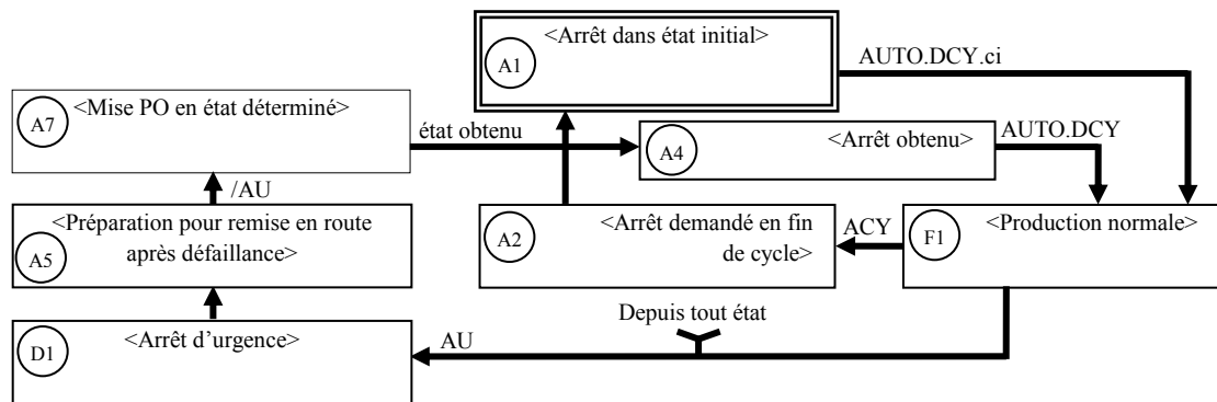
Figure (IV.12) : GEMMA d'une machine avec arrêt d'urgence et remise en route.
