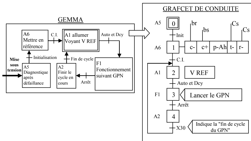
Figure (IV.17) : Elaboration de la Grafcet de conduite.
