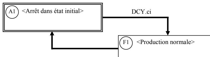
Figure (IV.6) : GEMMA minimal d'une machine semi-automatique.
