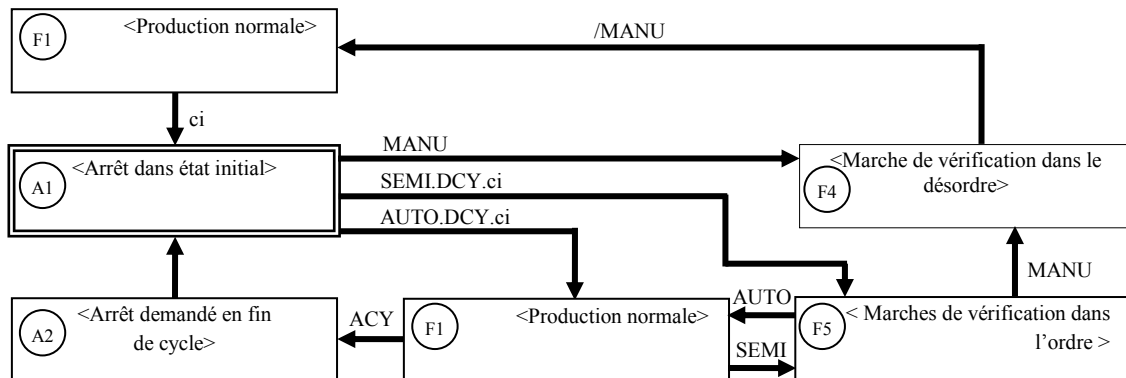
Figure (IV.15) : GEMMA d'une machine avec marches de vérification dans le désordre et dans l'ordre.
