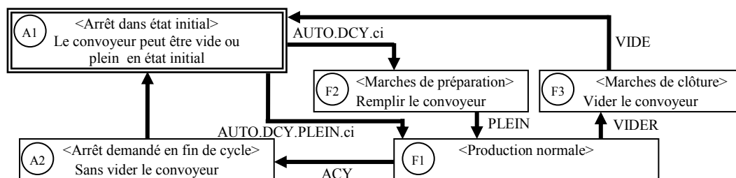
Figure (IV.9) : GEMMA d'une machine exigeant une marche de préparation et une marche de clôture.
