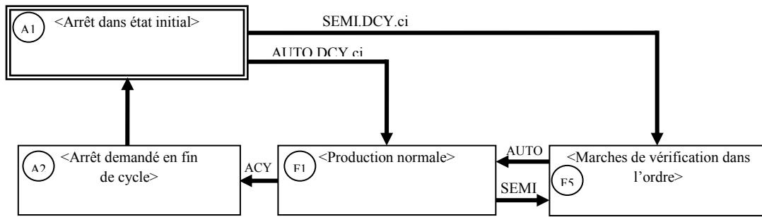
Figure (IV.14) : GEMMA d'une machine avec marches de vérification dans l'ordre.
