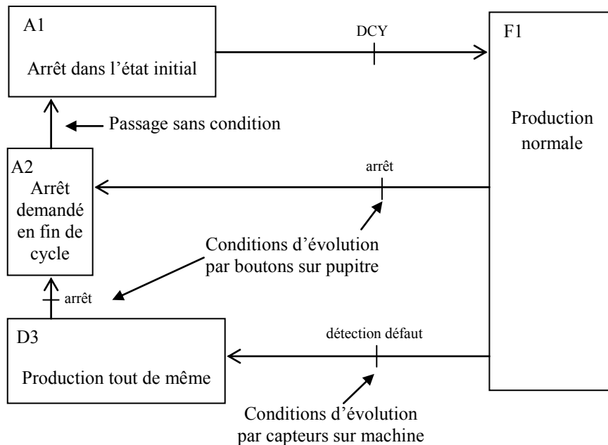
Figure (IV.5) : Conditions d'évolution entre modes marches / arrêts.
