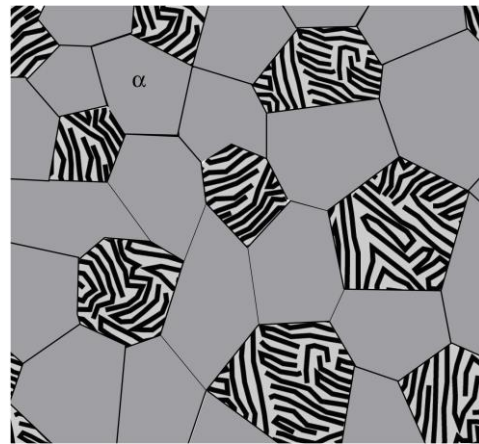
Figure 2 : Alliage hypoeutectique
