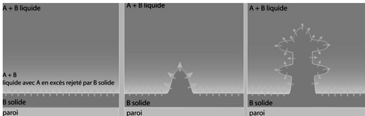
Figure 4 : Apparition de dendrite au contact de la paroi
