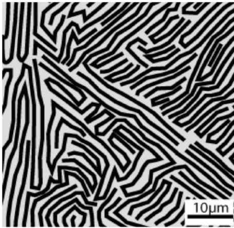
Figure 1 : aspect d'un alliage eutectique
