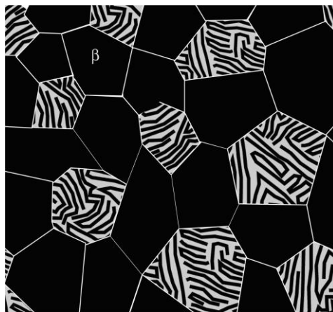
Figure 3 : Alliage hypereutectique
