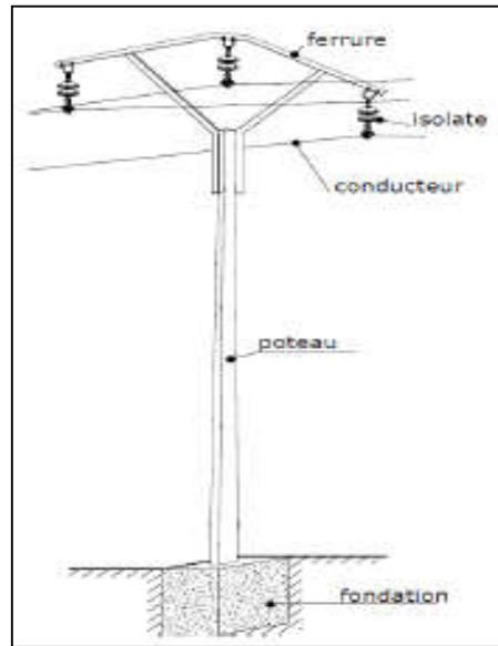
Figure 2.1: Les principaux composants des lignes aériennes
