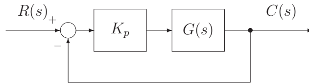
FIG. 7.2 – Contrôleur proportionnel dans un système.
