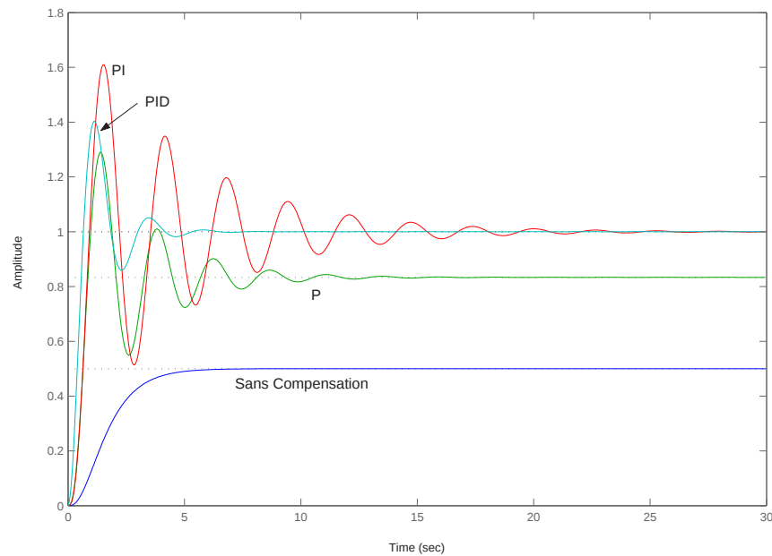
FIG. 7.6 – Simulation des réponses des compensateurs.
