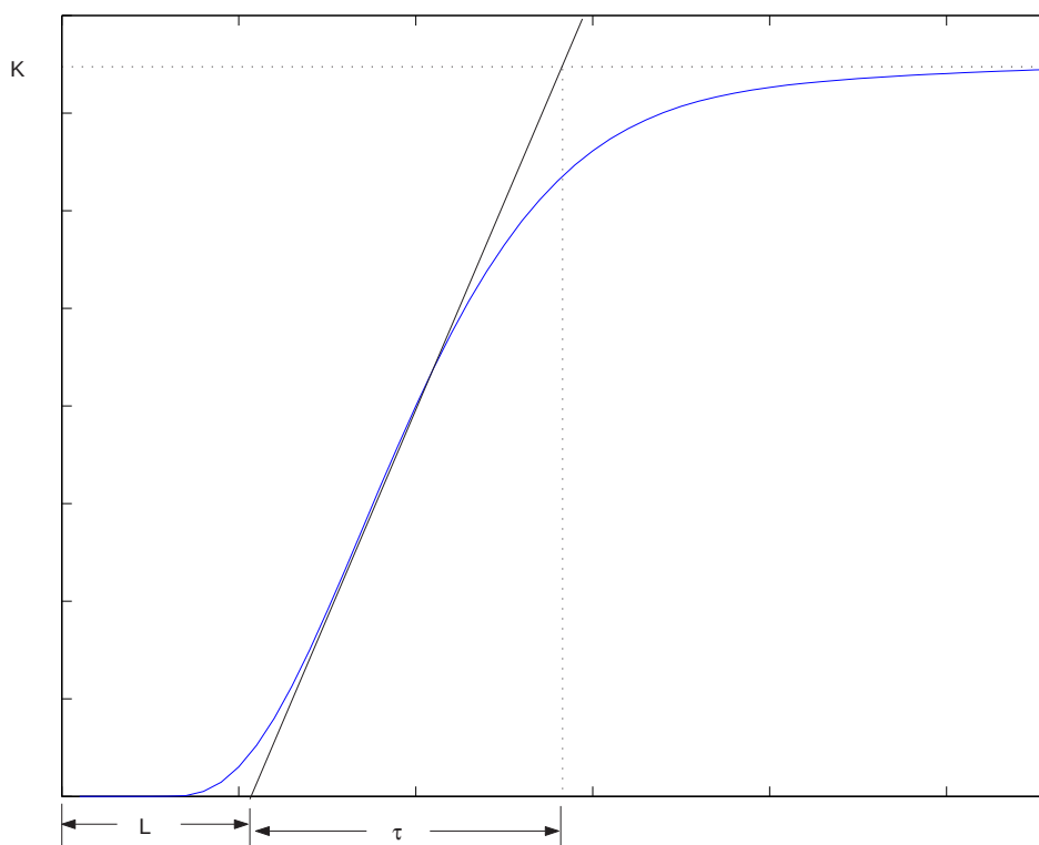
FIG. 7.3 – Réponse d'un système: courbe de réaction
