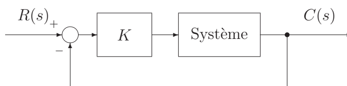
FIG. 7.4 – Système sous étude: Ziegler-Nichols.
