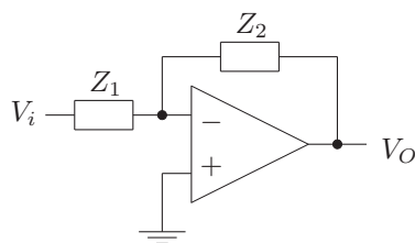
FIG. 7.7 – Ampli-op comme amplificateur avec feedback négatif
