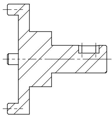
COUPE A-A
