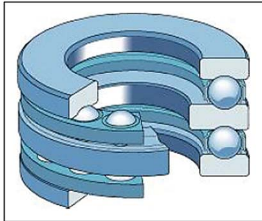
Figure 4.18. Butées à billes à double effet. [1,5,6]
