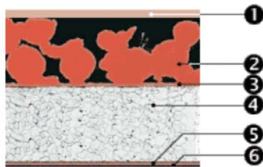
Figure. 4.4. Constituants du coussinet composite: 1 Polytetrafluorethylene (PTFE), 2 Bronze/étain ou Bronze/plomb, 3 Couche de liaison (cuivre), 4 Support en acier, ( 5 Couche de cuivre 6 Couche d'étain, Protection du support en acier).
