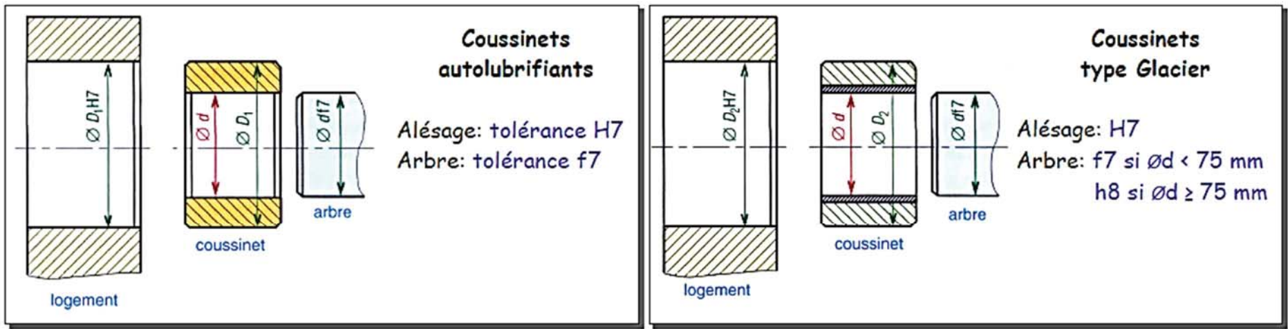
Figure 4.9. Ajustements sur coussinets. [5,6]
