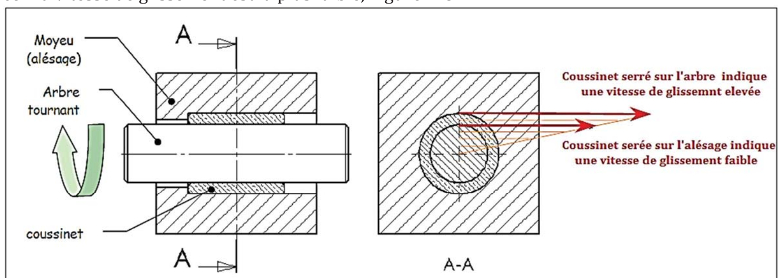
Figure. 4.8. Instructions de montage des coussinets. [5,6]
