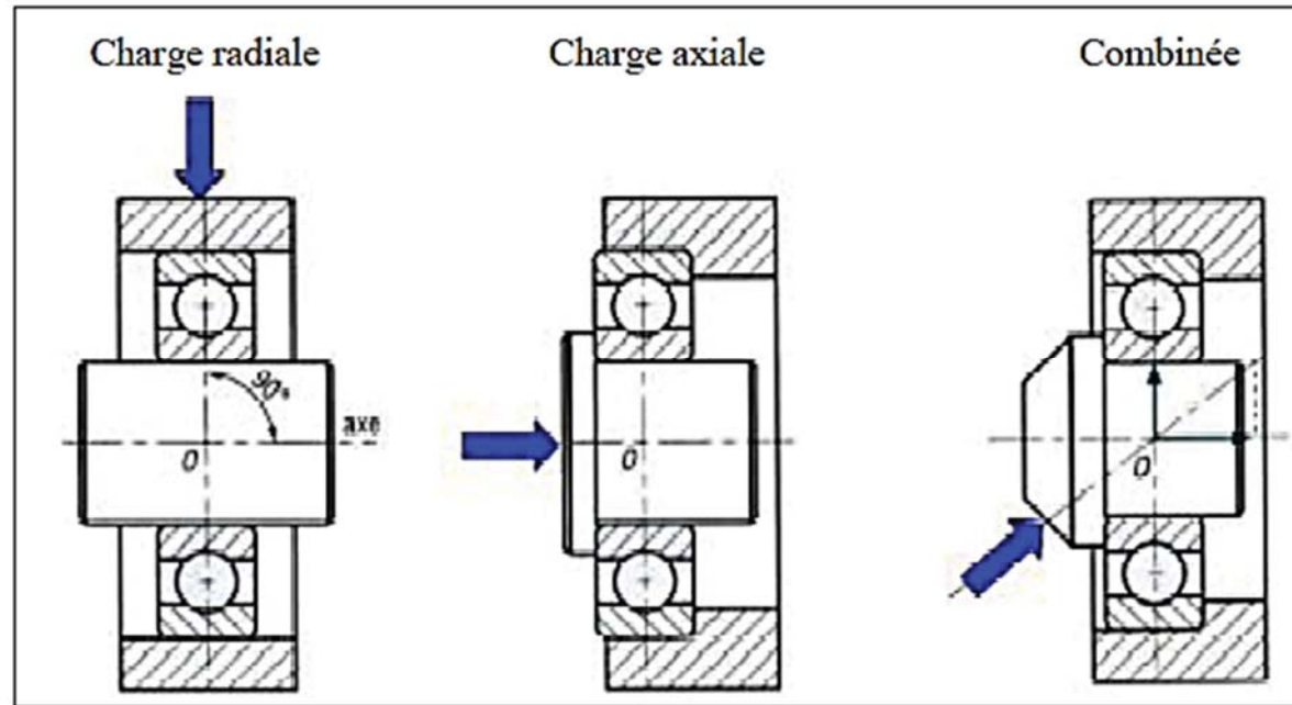
Figure. 4.23. Charges supportées par un roulement. [1,5,6]
