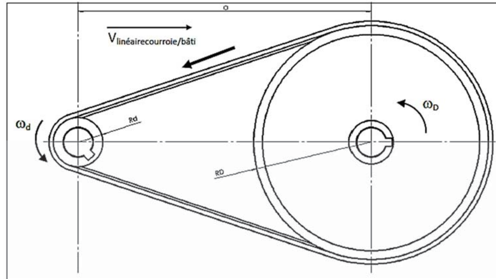
Figure. 4.24. Mécanisme de transmission par courroie. [1,5,6]
