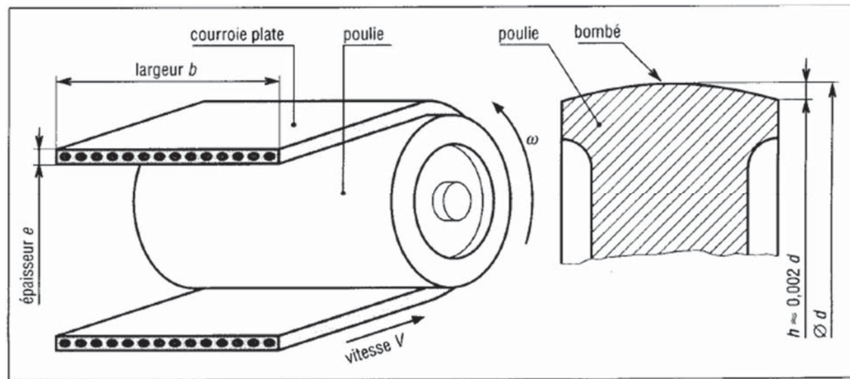
Figure. 4.25. Mécanisme de transmission par courroie plate. [1,5,6]
