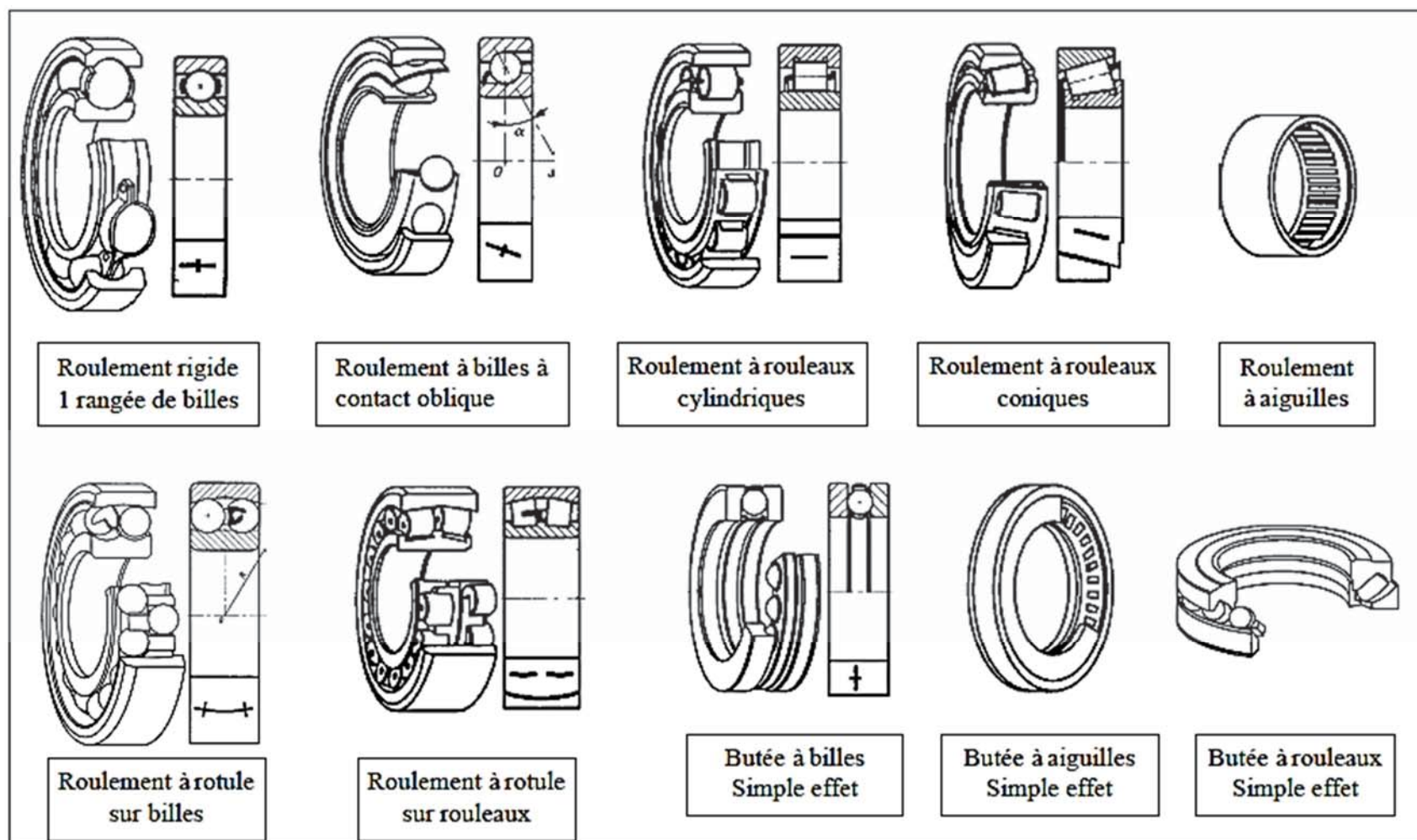
Figure .4.22. Symboles des roulements. [1,5,6]
