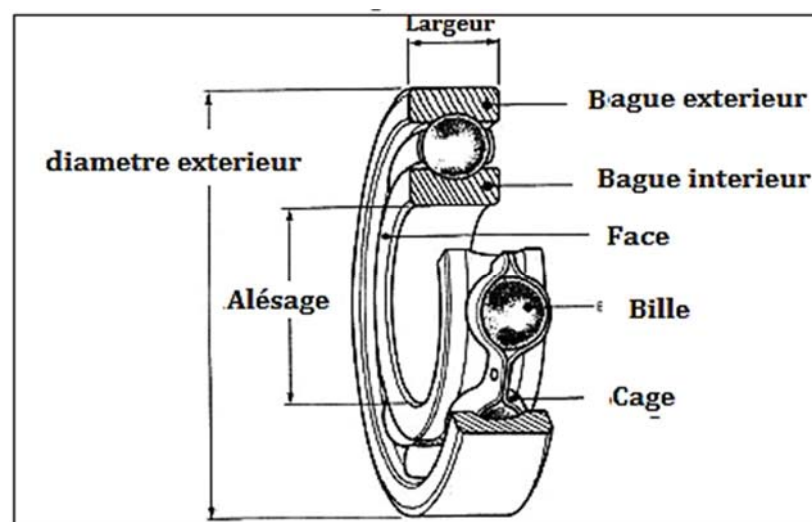
Figure. 4.10. Principaux éléments constitutifs d'un roulement. [1,5,6]
