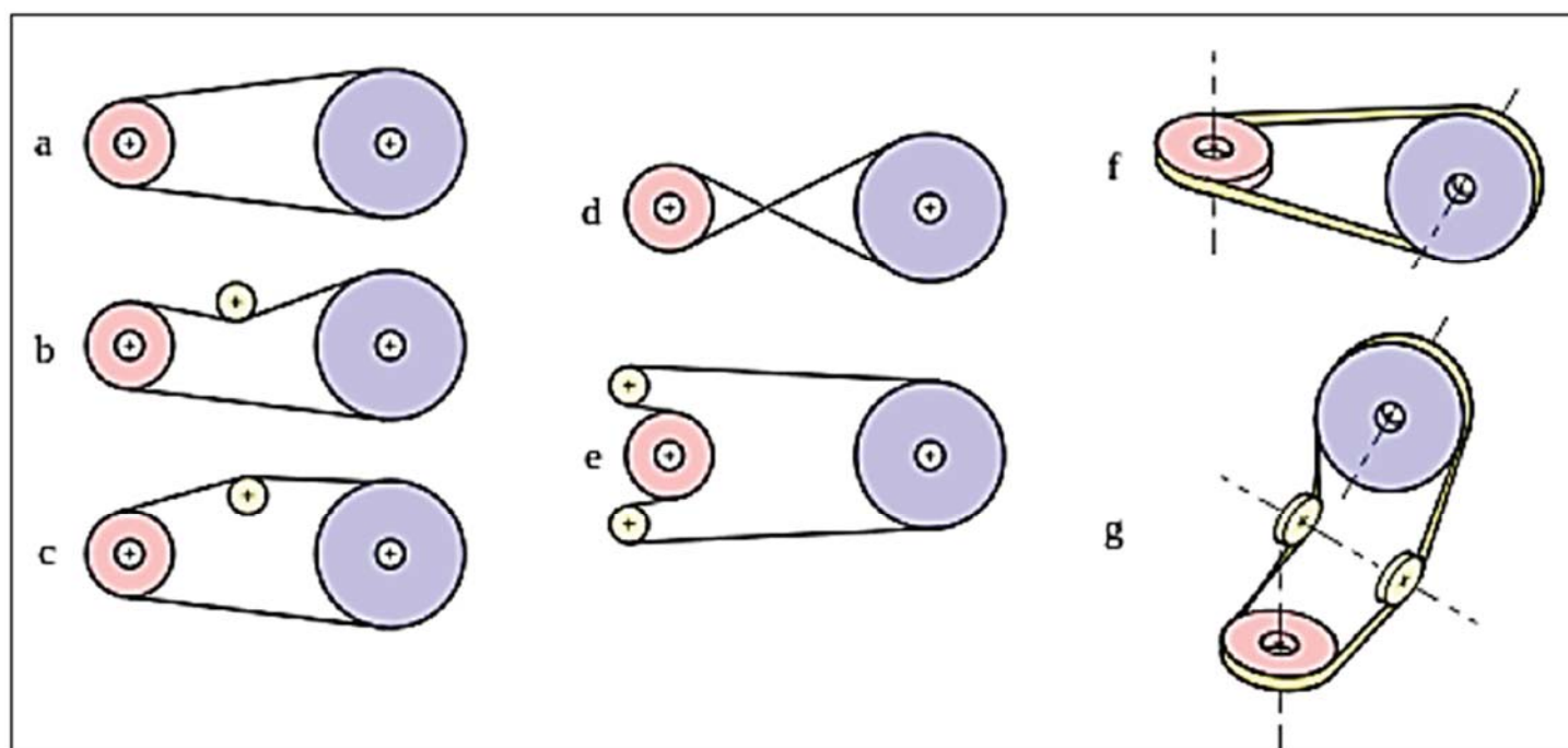
Figure. 4.28. Types de montage des courroies. [1,5,6]
