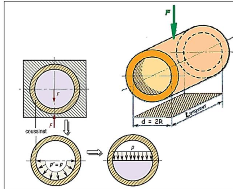
Figure. 4.6. Répartition des charges sur un palier. [1]
