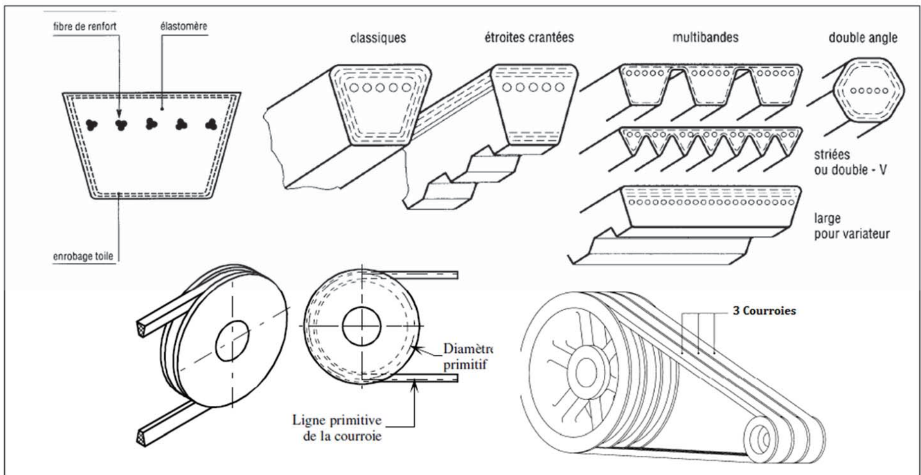
Figure. 4.26. Mécanisme de transmission par courroie trapézoïdale. [1,5,6]
