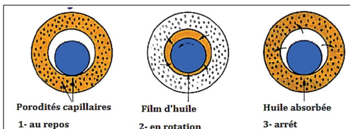
Figure 4.2. Paliers avec système autolubrification. [5,6]
