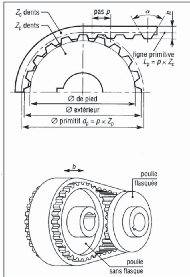
Figure. 4.27. Mécanisme de transmission par courroie crantée. [1,5,6]
