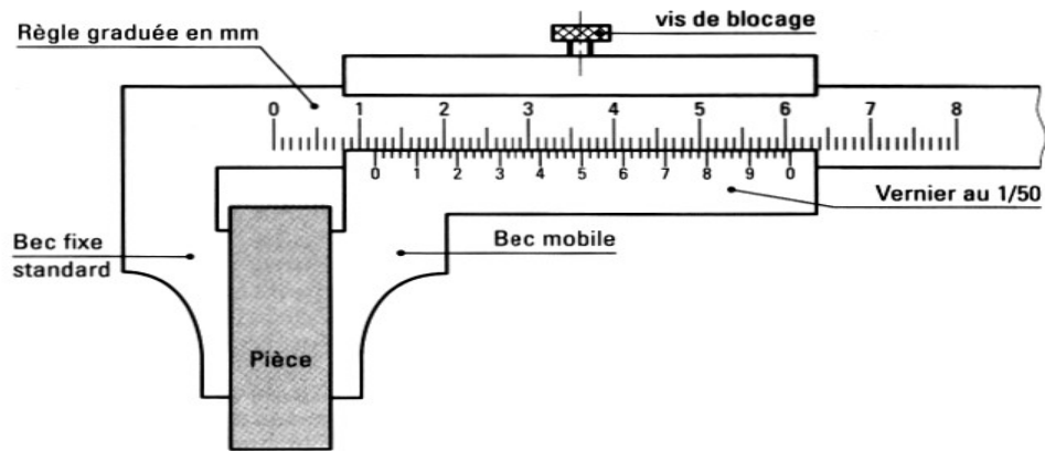
Fig.1 : Pied à coulisse universel (à becs)
