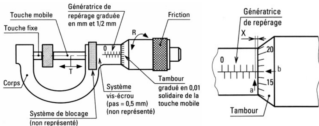
Fig.1 : Micromètre (Palmer)
