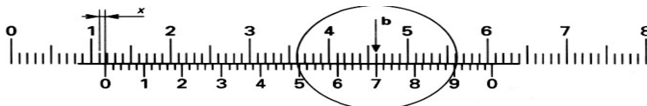
Fig.2 : Mesure au Pied à coulisse
