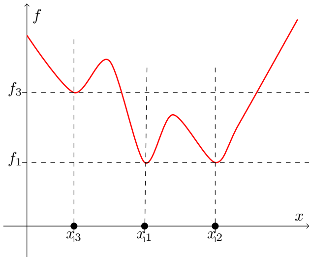
Figure 1 – Optimum local et global.
