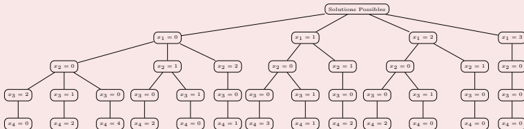
Figure 8 – Solutions possibles de l'exemple de sac à dos.
