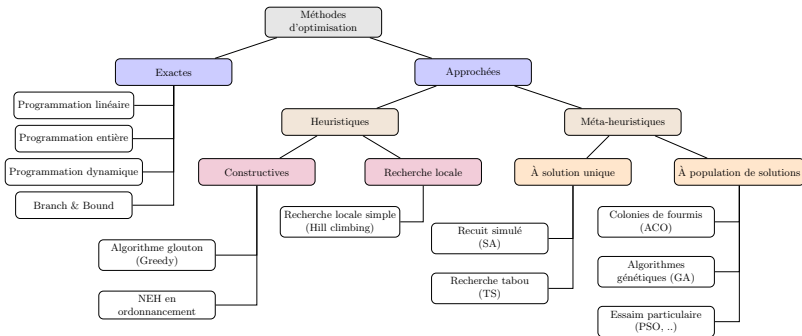
Figure 7 – Taxonomie des méthodes de résolution de problème d'optimisation.
