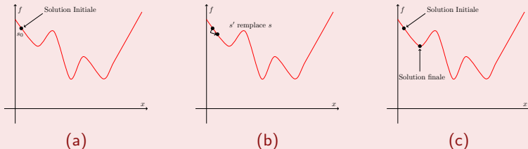
Figure 13 – Évolution d'une solution dans la méthode de descente
