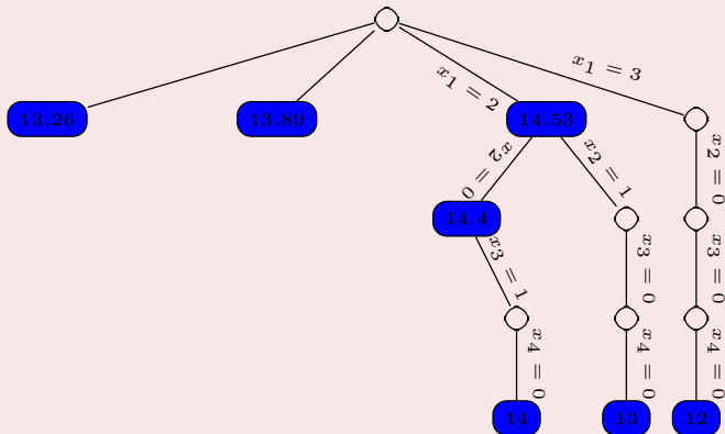
Figure 9 – Résolution de l'exemple de sac à dos par Branch & Bound.
