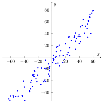
(b) Fonction discrète
