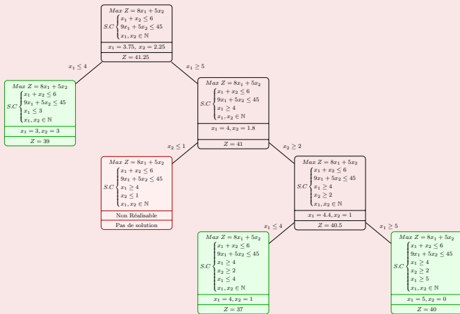
Figure 10 – Arborescence globale du problème par l'Éq. 8.
