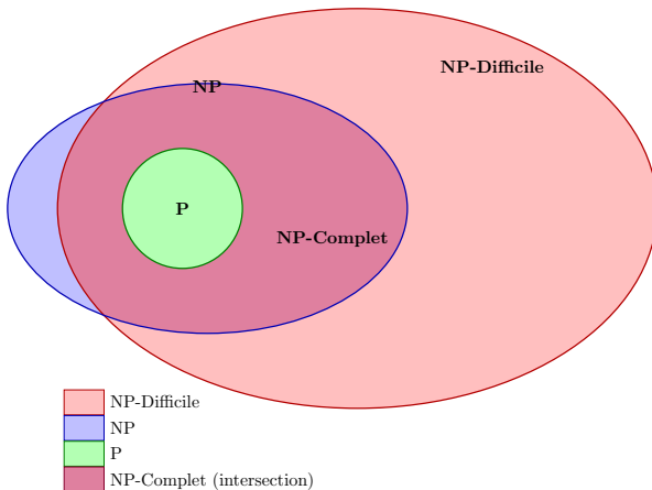
Figure 6 – Classes des Problèmes.
