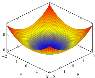
(a) Fonction continue
