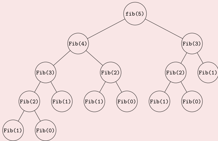
Figure 11 – Arbre d'appels naïf pour Fib(5) .
