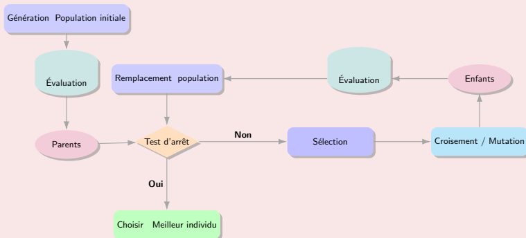
Figure 15 – Principe de l'algorithme génétique.
