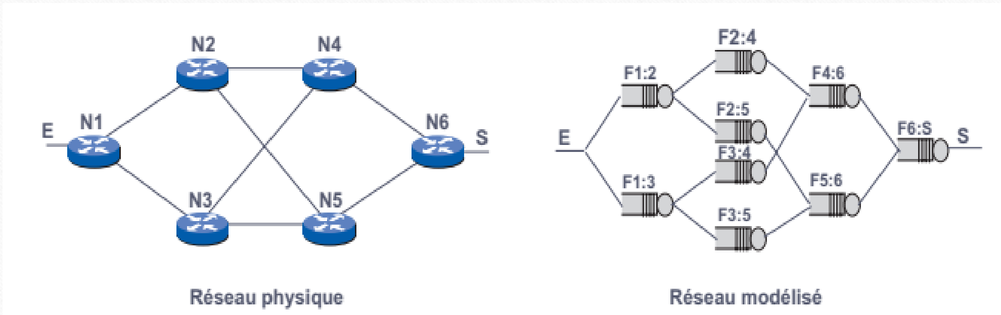
Figure 3.16 : Modélisation d'un réseau.
