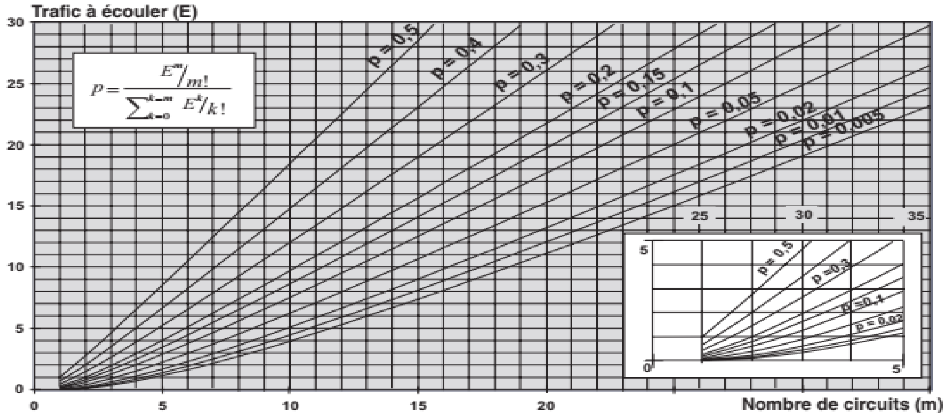
Figure 3.8 : Abaque d'Erlang (refus)
