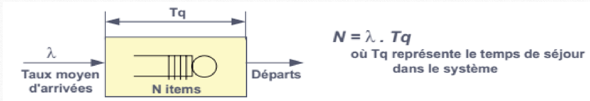
Figure 3.10 : Formule de Little.
