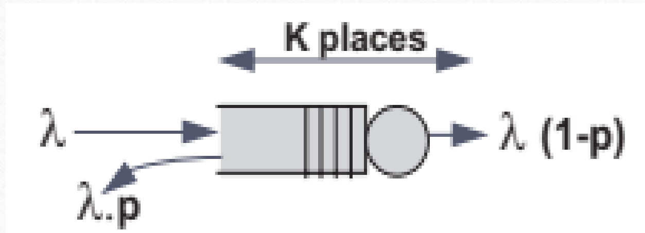
Figure 3.15 File d'attente à capacité limitée.
