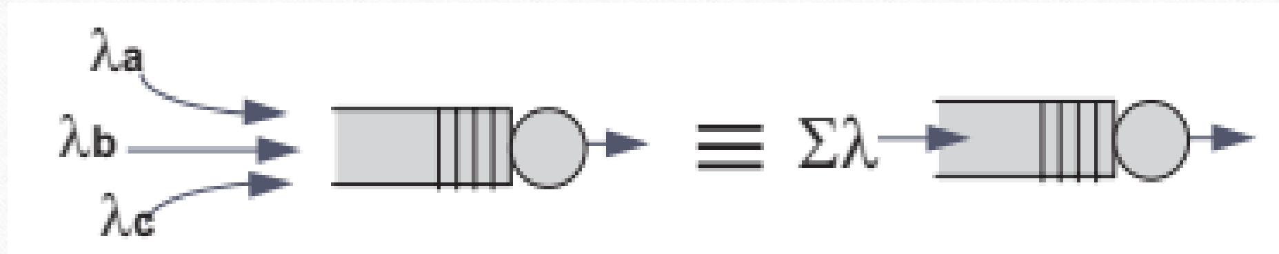
Figure 3.14 : File d'attente avec entrées multiples.
