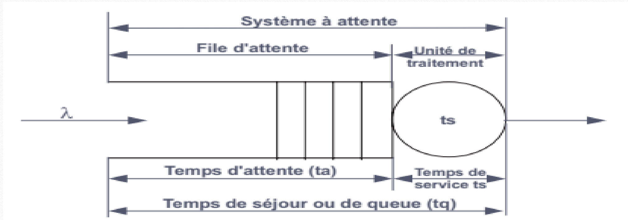
Figure 3.11 : Modélisation d'une file M/M/1/∞.
