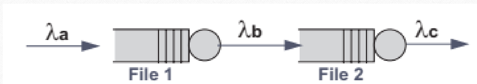
Figure 3.12 : Réseau ouvert de files d'attente en série.
