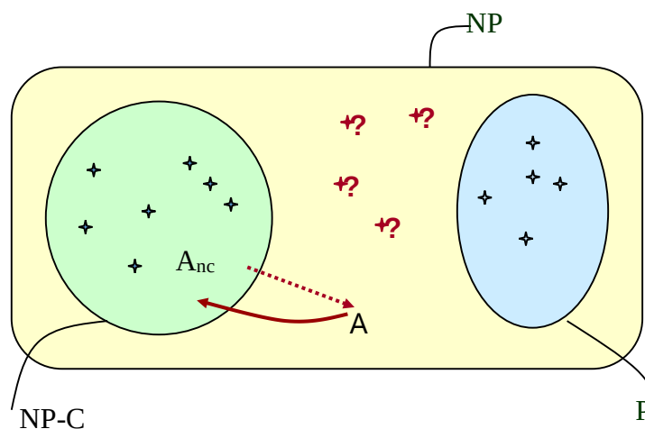
Figure II. 3. Représentation d'une réduction polynomiale.
