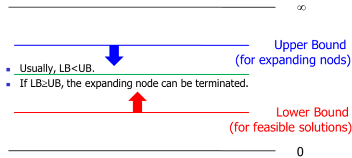
Figure V.2. Choix des bornes.
