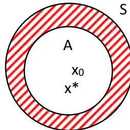
Figure III.1. Espace de recherche et solutions admissibles.
