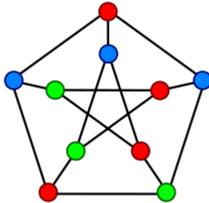
Figure III.7. Représentation d'une solution du problème 3-coloration.
