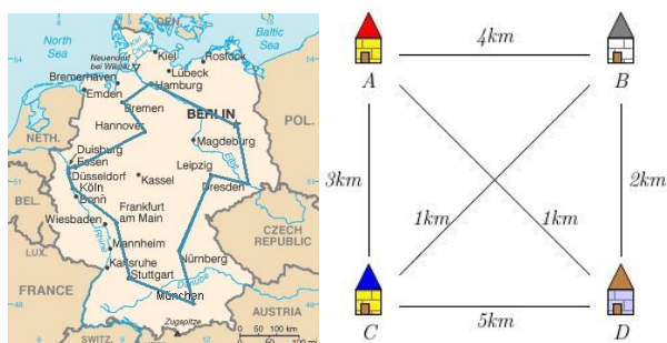
Figure III.5. Exemple de TSP.
