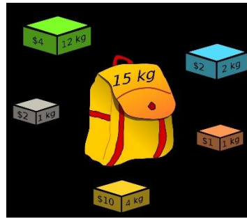
Figure III.4. Exemple de KSP.
