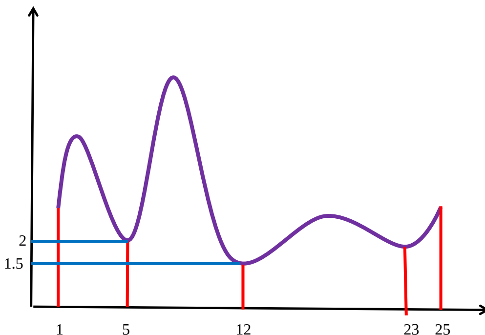
Figure III.2. Représentation graphique de la fonction f de l'exemple 1.
