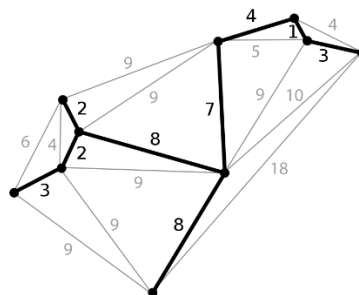
Figure III.8. Représentation de l'arbre couvrant minimal dans un graphe.
