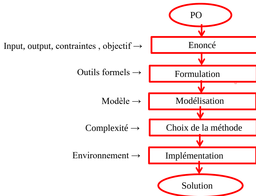
Figure III.3. Processus de résolution d'un PO.
