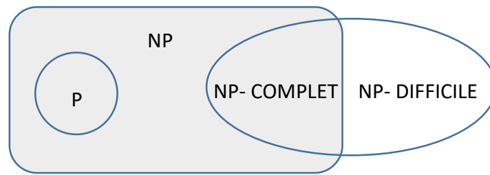
Figure II. 2. Classes de problèmes.
