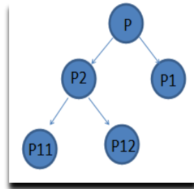
Figure V.1. Schéma de séparation.
