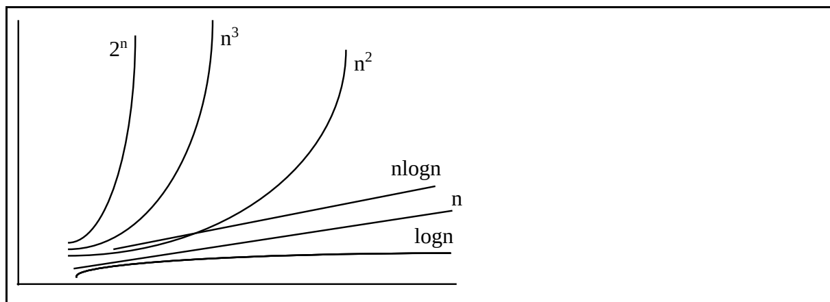
Figure II. 1. Allure de quelques courbes.
