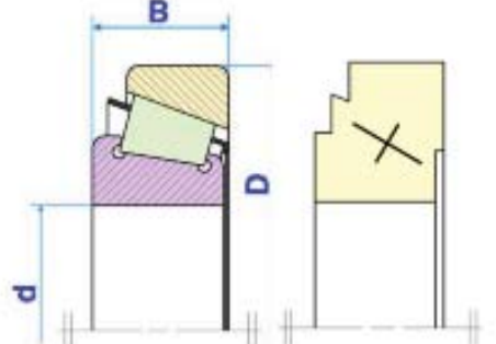
مدحرجات ذات دحاريج مخروطية
