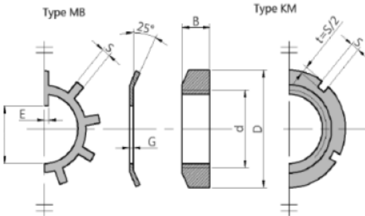
صامولة محززة
