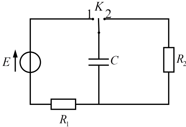
الشكل 4. دارة تجربة شحن وتفريغ مكثفة
