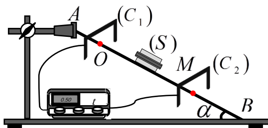
الشكل 9. حركة جسم صلب فوق مستوي مائل
