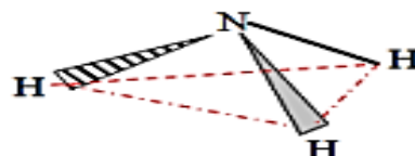
جزيء النشادر
