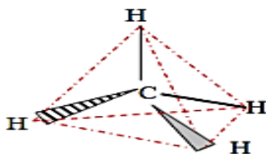
جزيء الميثان
